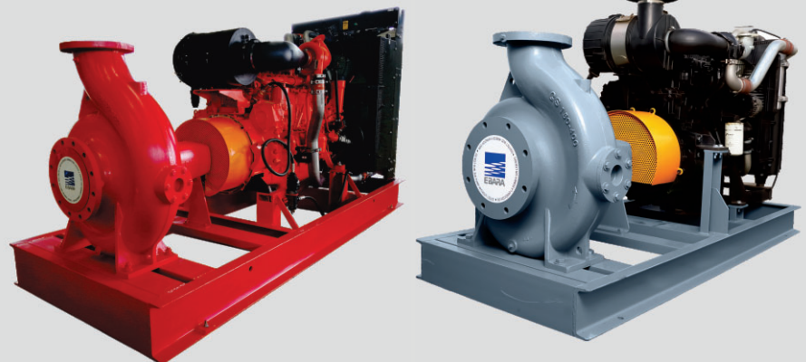
Flanges ANSI 16bar (ANSI B 16.1) Opcional DIN 16bar (EN PN16)
