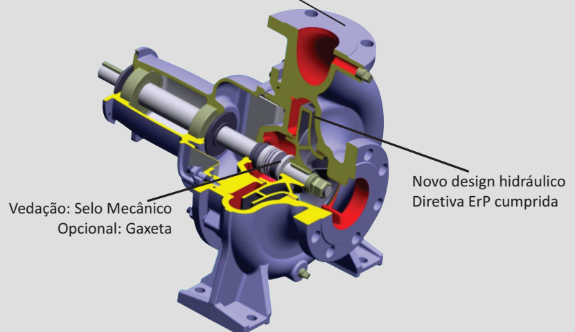
Flanges ANSI 16bar (ANSI B 16.1) Opcional DIN 16bar (EN PN16)
