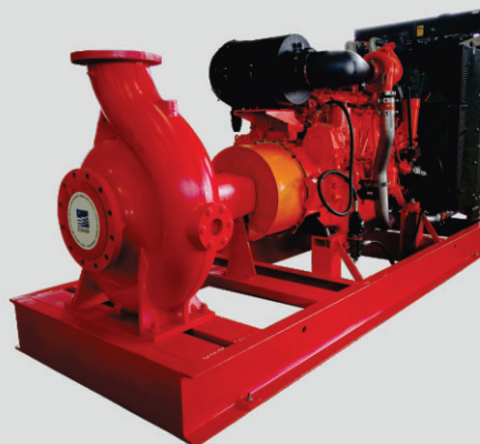
Flanges ANSI 16bar (ANSI B 16.1) Opcional DIN 16bar (EN PN16)
